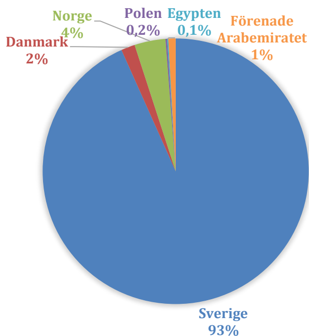
Figur 8 Fördelning av klimatmissioner på samtliga verksamhetsländer år 2017 (ton CO 2 e).
