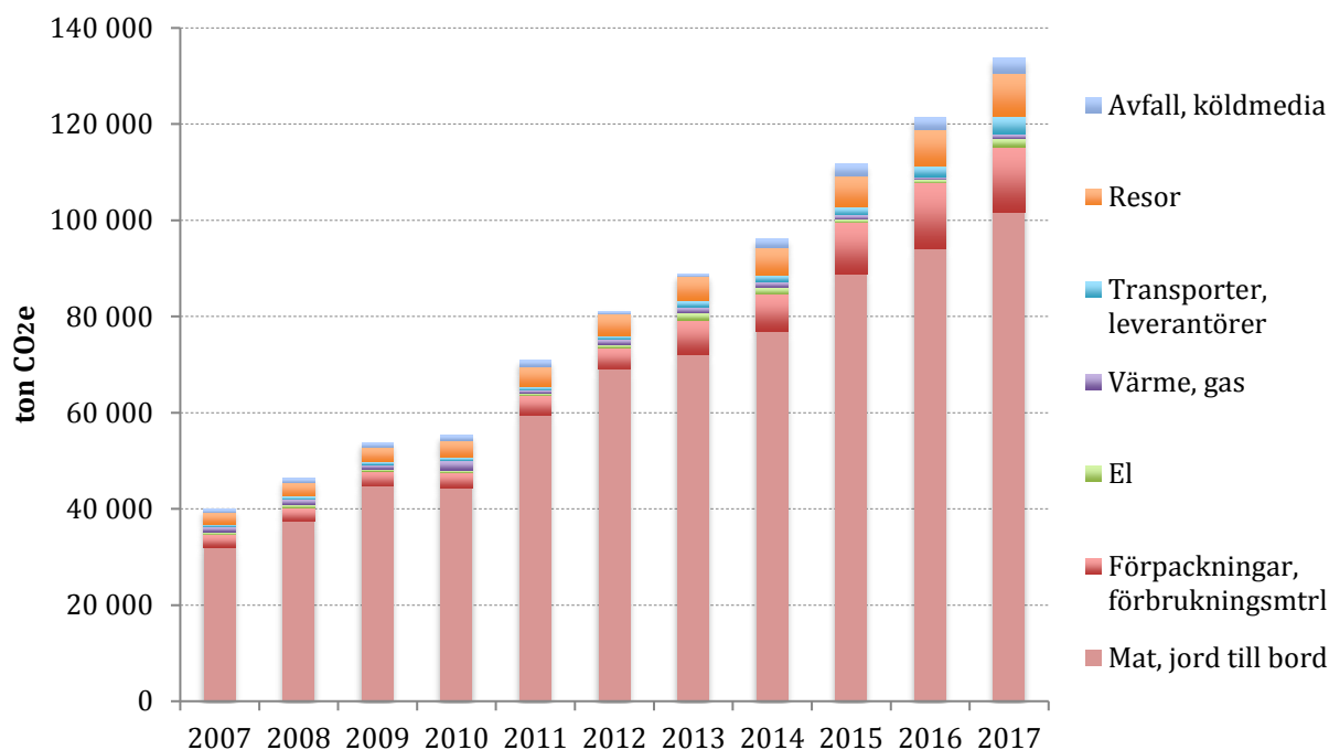
Figur 2 MAX klimatfotavtryck sett i ett livscykelperspektiv, dvs från odling av foder och uppfödning till tillagning i restaurang och vidare till gästens resor och hantering av avfall. 4
