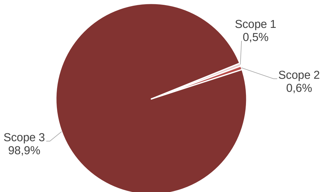
Figur 5 MAX klimatfotavtryck fördelat på scope 1, 2 och 3 för år 2017 (ton CO 2e ).
