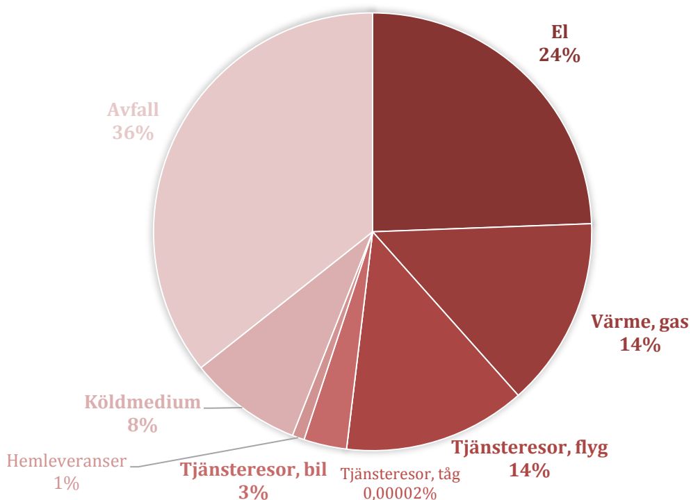
Figur 6 MAX klimatfotavtryck av den egna verksamheten såsom el, värme, kyla, köldmedia för restauranger och kontor samt tjänsteresor år 2017 (ton CO 2e ).
