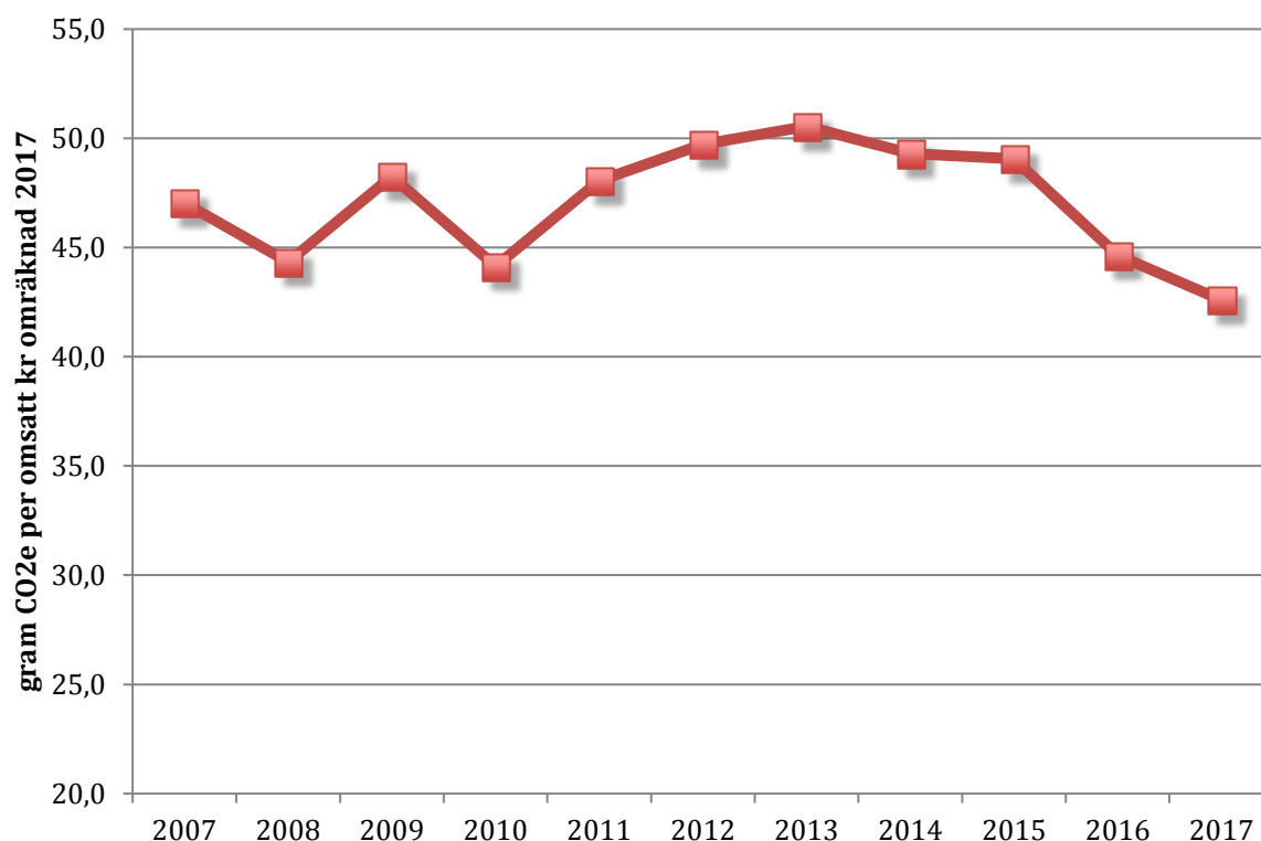
Figur 3 MAX klimatfotavtryck i antal gram CO 2 e från jord till bord och jord igen, fördelat per omsatt krona mellan år 2007-2017. 6
