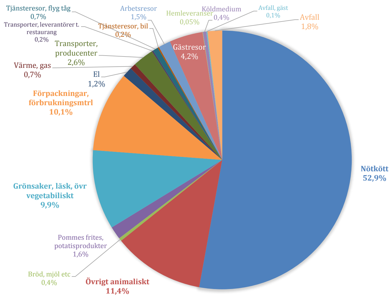
Figur 4 MAX klimatfotavtryck över hela livsrygeln fördelat på olika ingredienser respektive aktiviteter för år 2017 (ton CO 2e ).
